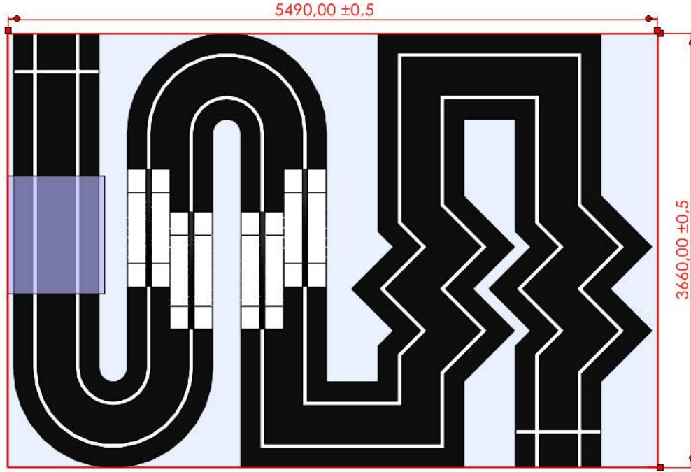
Şekil 4. Yarışma pisti ölçüsü
