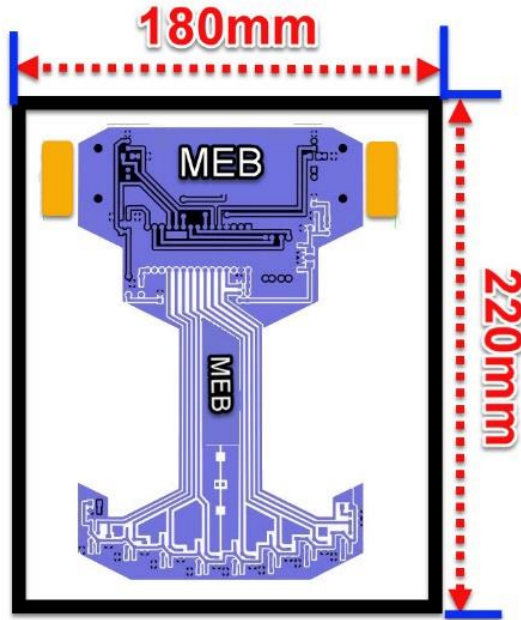
Şekil 1. Temel seviye robot ölçüleri
