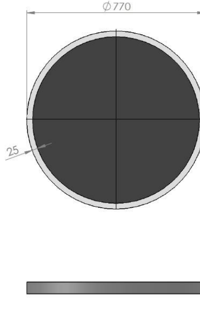
Şekil 1: Mini Sumo Robot Dohyo Ölçüleri (mm)
