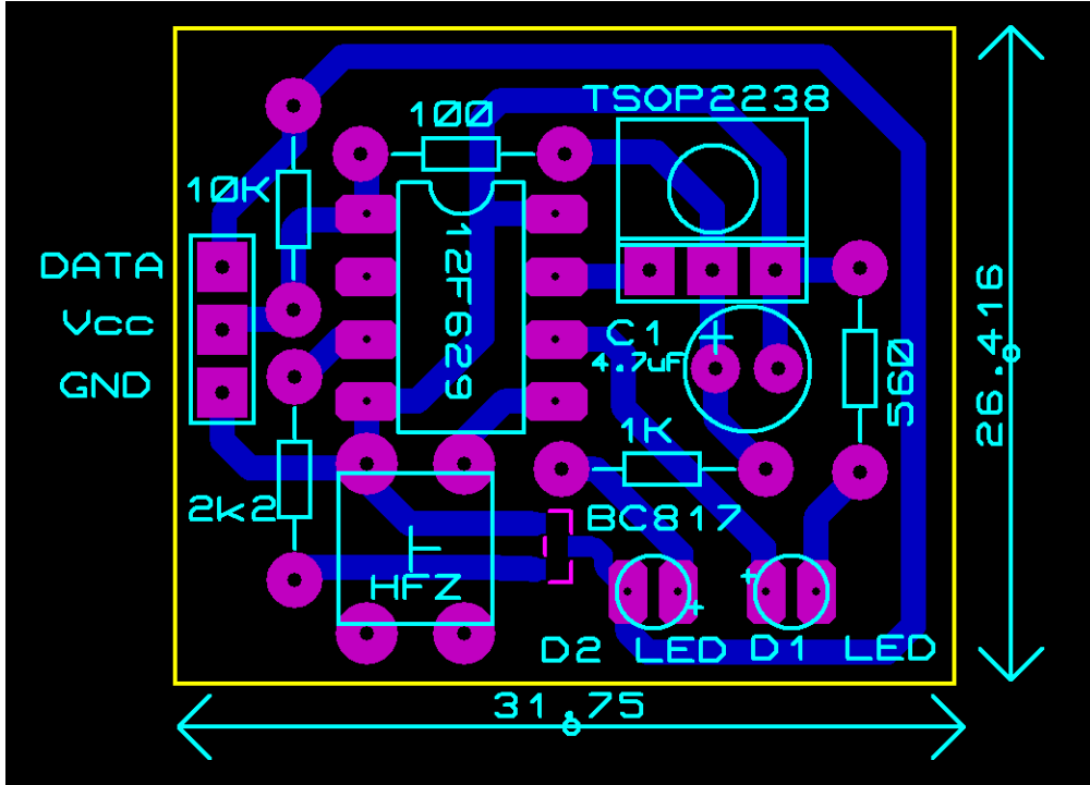
Şekil 2 : Start Modülü Baskı Devre Şeması START MODÜLÜNÜN ÇALIŞMASI
